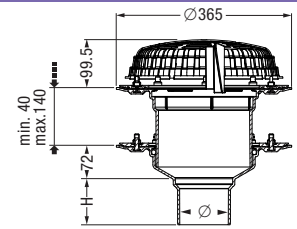
Размеры монтажа \varnothing 227 мм
