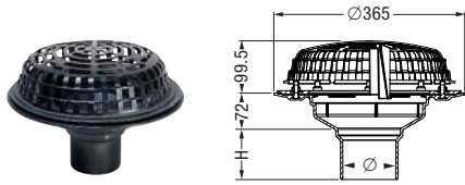
Размеры монтажа \varnothing 227 мм
