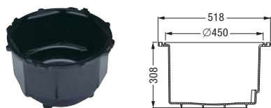
Корпус из полиэтилена
