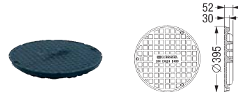
Крышка из полимера
