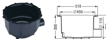
Корпус из полиэтилена
