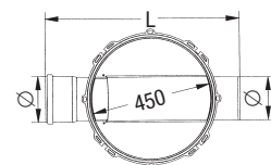
Корпус из полиэтилена с открытыми лотками
