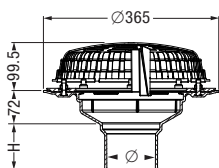
Размеры монтажа \varnothing 227 мм
